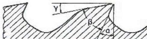
Εικ. 7.4 Γωνίες κοπής
