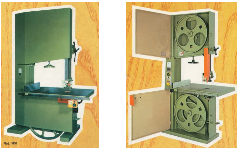
Εικ. 7.2 Ταινιοπρίονο
