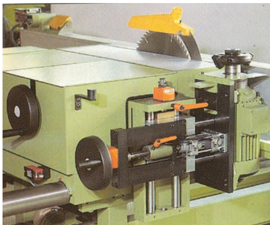
Εικ. 7.3 Δισκοπρίονο
